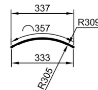
Стекло в вогнутую рамку с четвертью Нстекла=594мм (794мм)
