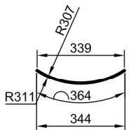
Стекло в выпуклую рамку с четвертью Нстекла=594мм (794мм)
